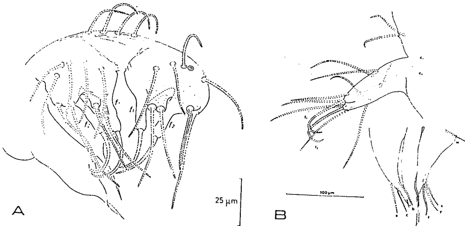
Fig. 4. - A. Eukoenia pauli Condé, d'après Condé (1979). B. Eukoenia pyrenaica (Hansen, 1926), de profil, les deuxième et troisième volets isolés, d'après Condé (1989). Explication des lettres comme sur les figures précédentes.
