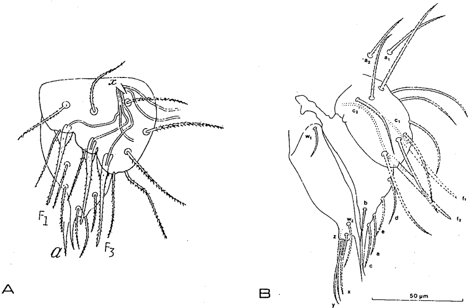
Fig. 2. - A. Prokoenenia millitorum Remy, lobes gauches des volets, d'après Remy (1950), légèrement modifié. a = point du 3 e volet ; F_1 - F_3 = fusules ; x = points où les canaux n'ont pu être suivis. B. Prokoenenia javanica Condé, volets de profil, d'après Condé (1990). Lettres comme sur la fig. 1, sauf a_1 , a_2 = phanères de la rangée antérieure ; a à e = phanères du 2 e volet ; w_1 , w_2 = dédoublement du w .
