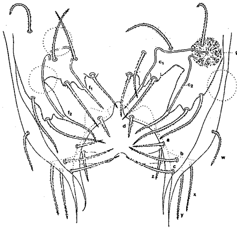
Fig. 1. - Eukoenenia mirabilis (Grassi), d'après Condé (1948), légèrement modifié. c_1 , c_2 = canaux évecteurs ; f_1 , f_2 = fusules ; g = acinus ; a à d = phanères ordinaires du 2 e volet ; w à z = phanères du 3 e volet.
